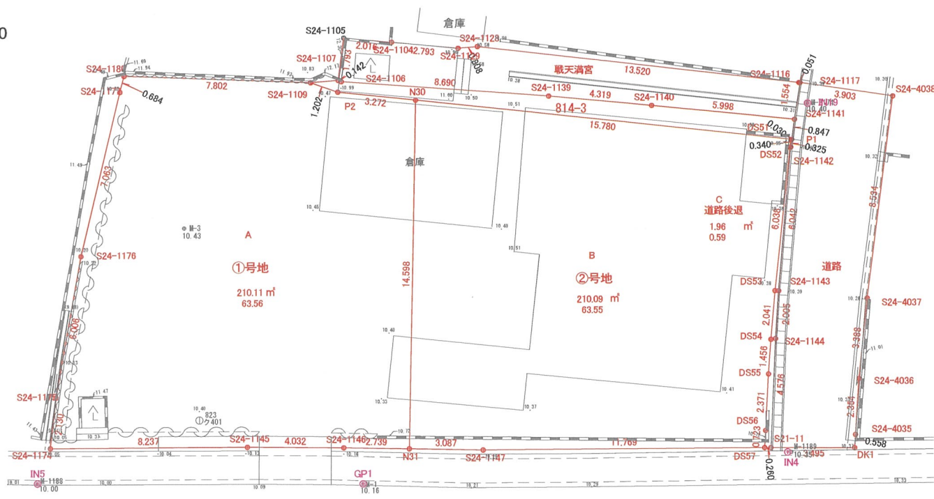
求積表
