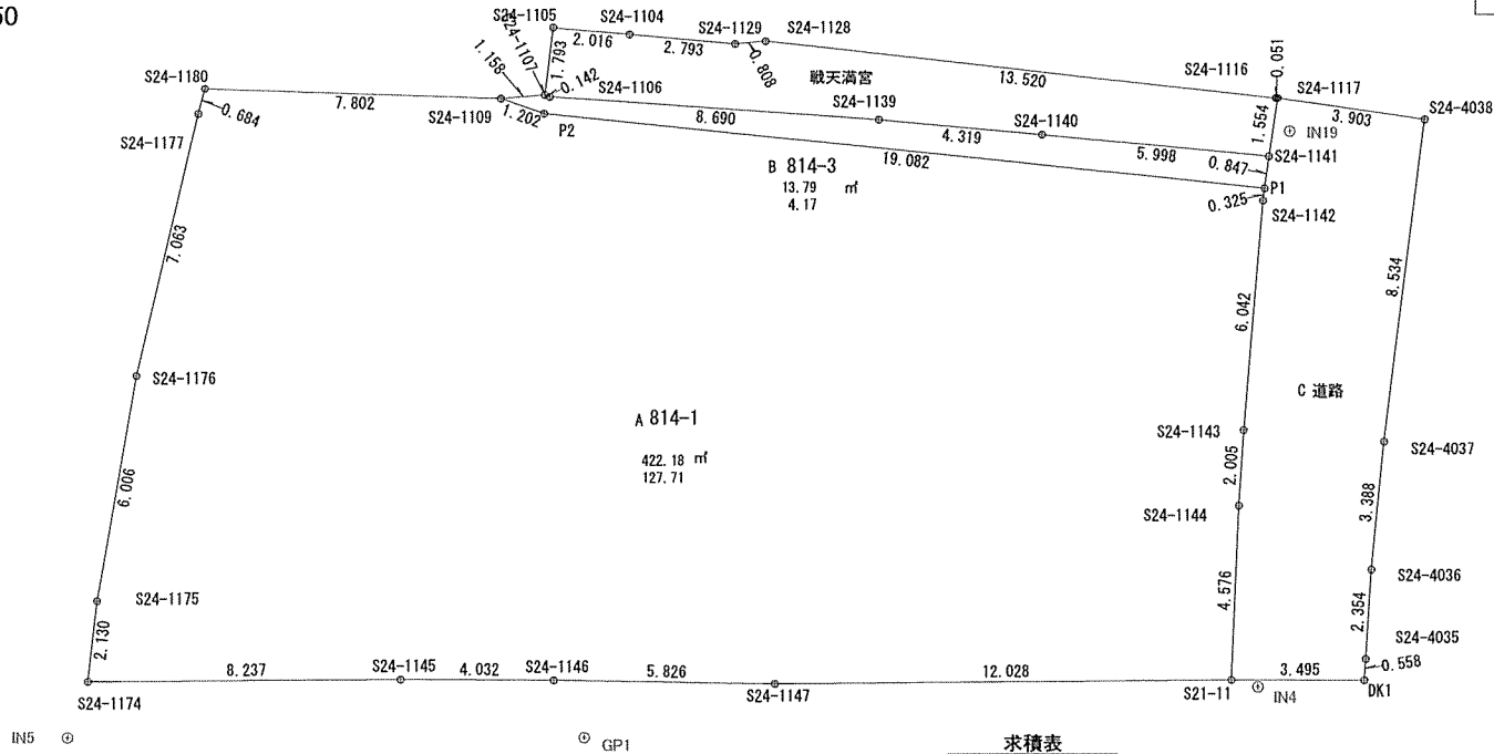
求積表
